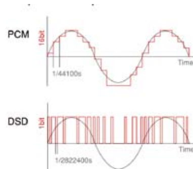
Samplingfrequenz bei PCM und DSD im Vergleich
