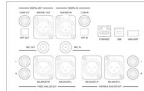
Analoge & digitale Ein- und Ausgänge
