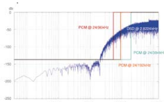
Signal / Rauschabstand bei PCM und DSD im Vergleich
